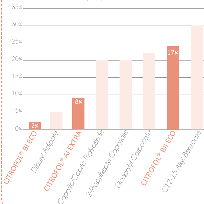
% d'émoullient nécessaire pour solubiliser 1% de UVINUL® T 150 Ethylhexyl Triazone
