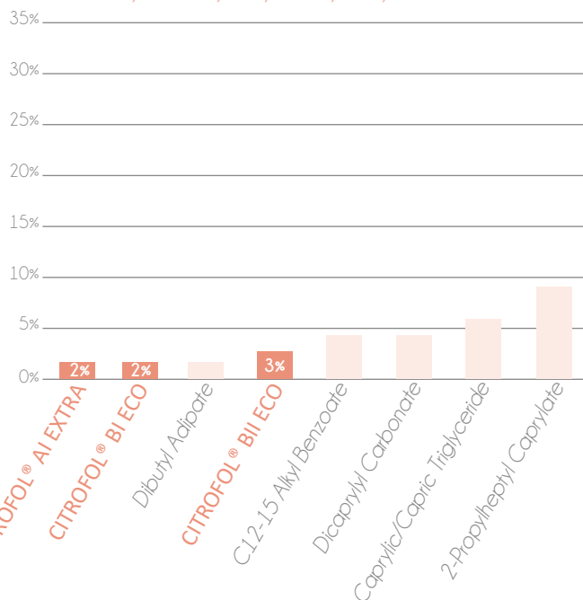
% d'émoullient nécessaire pour solubiliser 1% de UVINUL® A PLUS GRANULAR Diethylamino Hydroxybenzoyl Hexyl Benzoate
